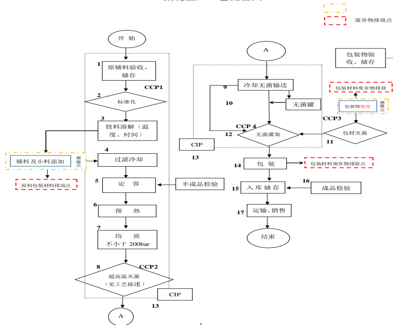
图 3-4 复合蛋白饮料工艺流程图
