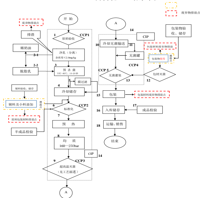
图 3-3 调制乳工艺流程图
